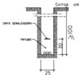
TERRENO TIPO I (Terreno de cultivo)
